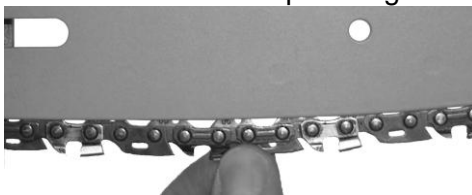
Korrekte Kettenspannung
