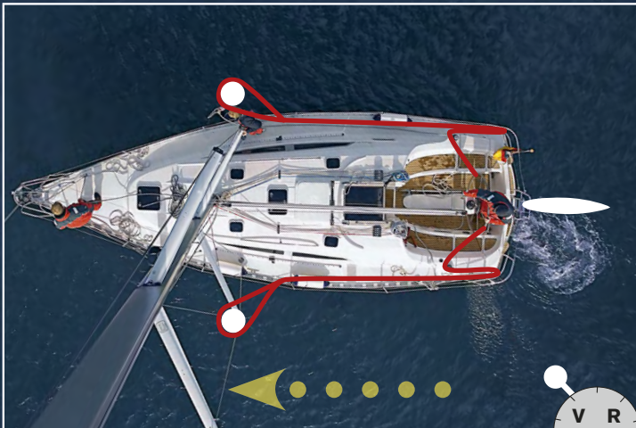
1 Sobald die Pfähle erreichbar sind, beide Mittelsprings festmachen. Die Yacht läuft währenddessen langsam in die Box.
